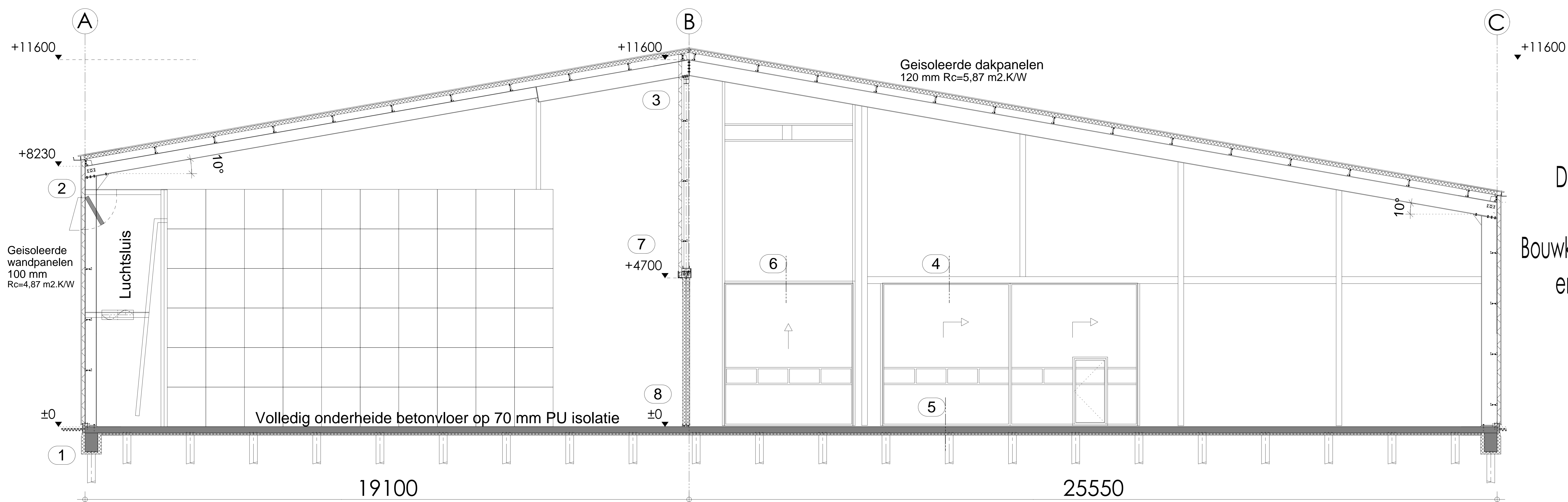
Doorsnede A-A
